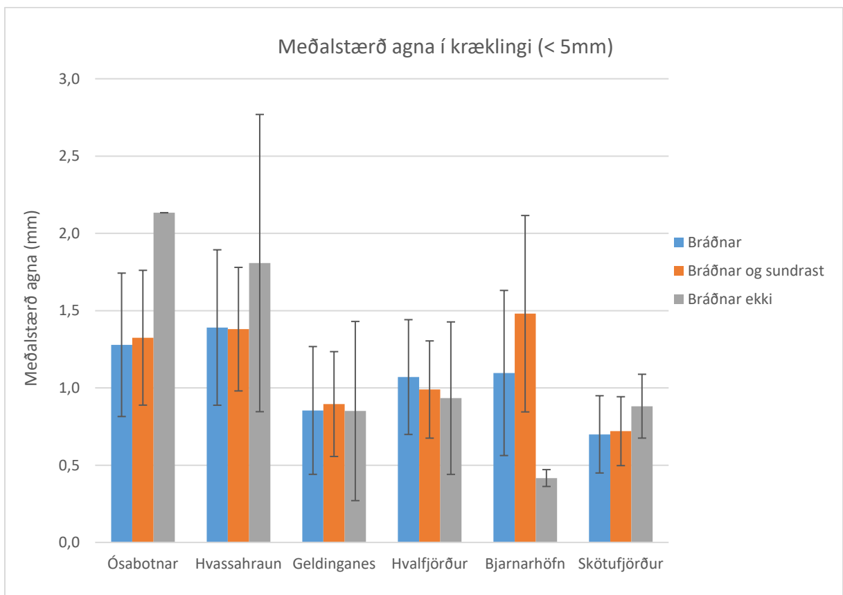
Mynd 5. Samanburður á meðalstærð (mm) þeirra agna sem fundust í kræklingi á mismunandi stöðvum. Hvergi er um að ræða marktækan mun á milli stöðva á stærð agna sem bráðna (Einþátta ferveikagreining; F_{5,57} = 1,621 ; p = 0,169 )
