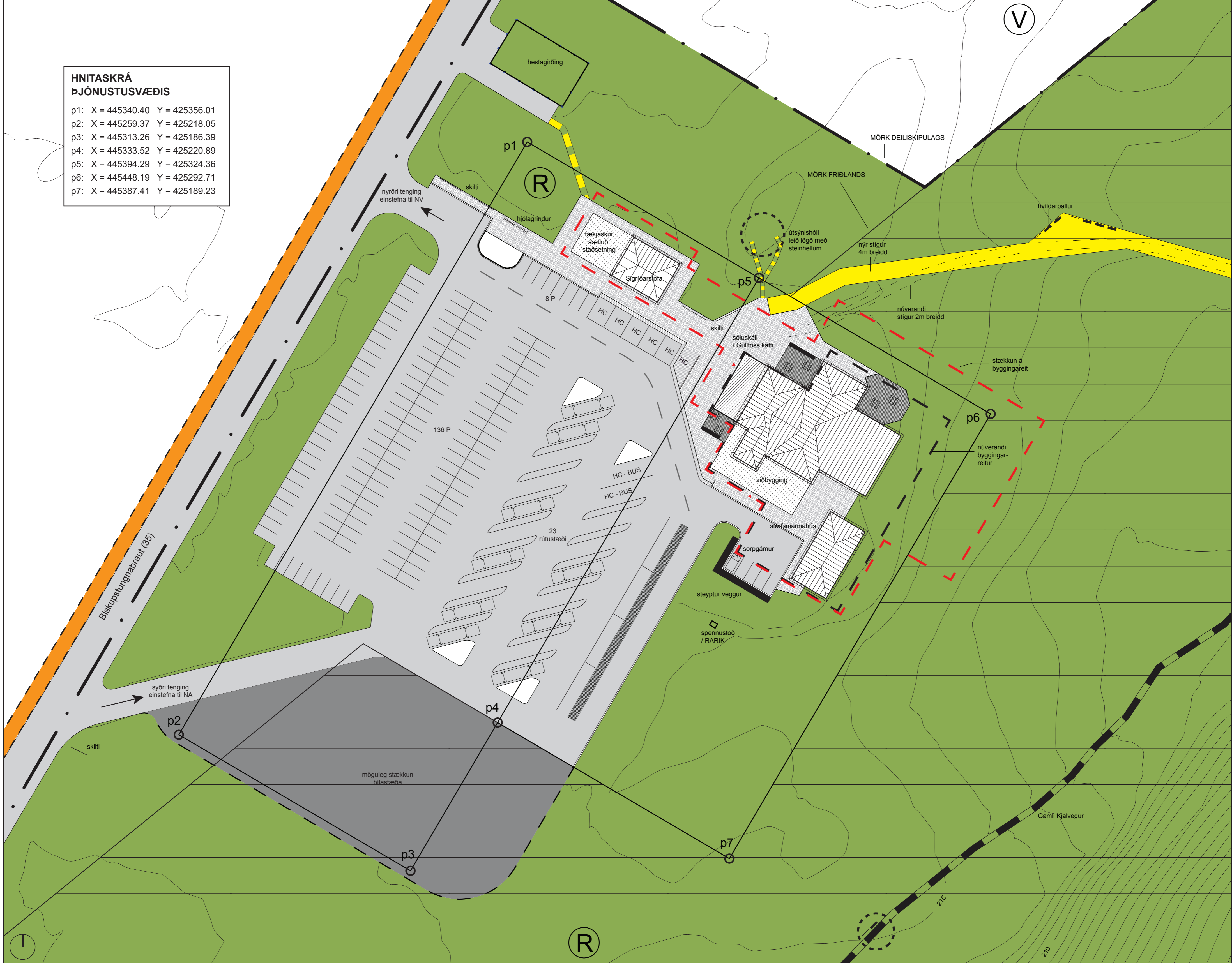
M1 - ferðþjónustuvæðið mkv. 1:500
